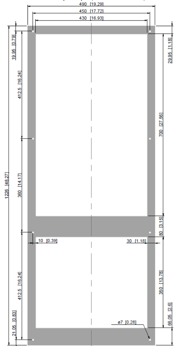
Монтажные размеры (внешний монтаж)
