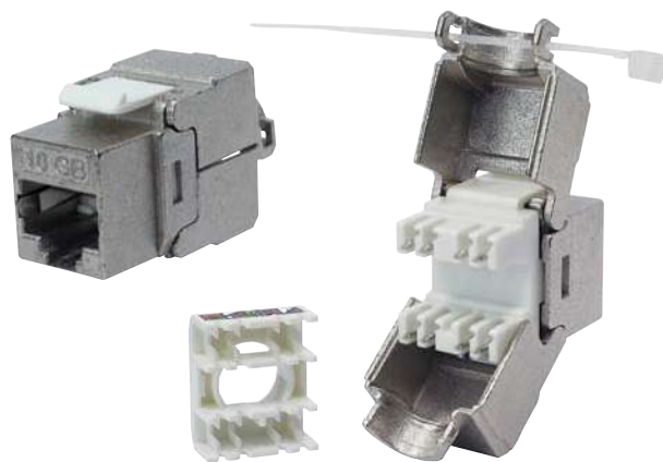
Keystone STP RJ45 категории 6 A – номер модели: T-SO-834-933
