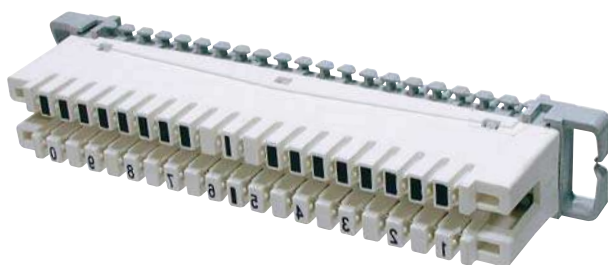
Плинт размыкаемый на 10 пар, 1-0, белый – номер модели: T-SO-870-500
