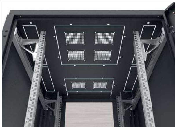
Верхняя панель шкафа
