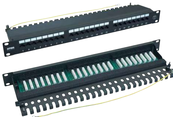
Патч-панель UTP 19" x 1 U, кат. 6, 24 порта черная с полкой и крышкой – номер модели: T-SO-806-120
