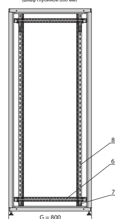
Вид сбоку (шкаф глубиной 800 мм)
