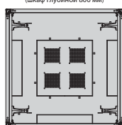
Разрез В-В (шкаф глубиной 800 мм)
