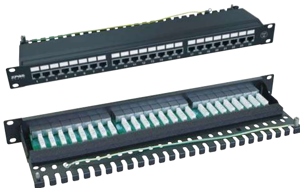
Патч-панель STP 19" x 1 U, кат. 5e, 24 порта черная с полкой и крышкой – номер модели: T-SO-805-526
