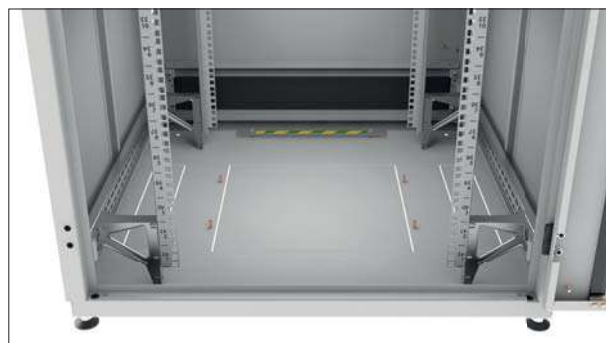
Нижняя панель шкафа. Задняя дверь оснащена панелью с щеточным кабельным вводом
