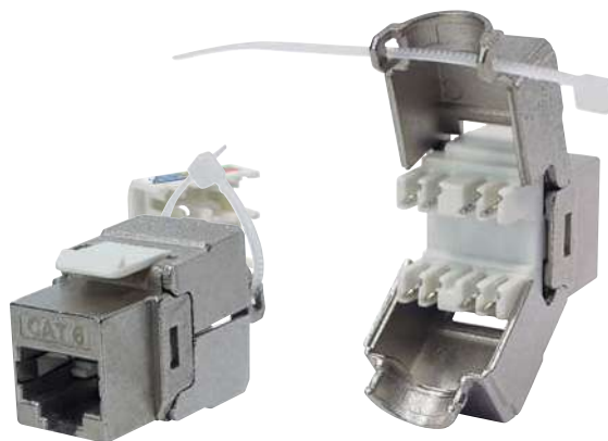
Keystone STP RJ45 категории 6 – номер модели: T-SO-832-924
