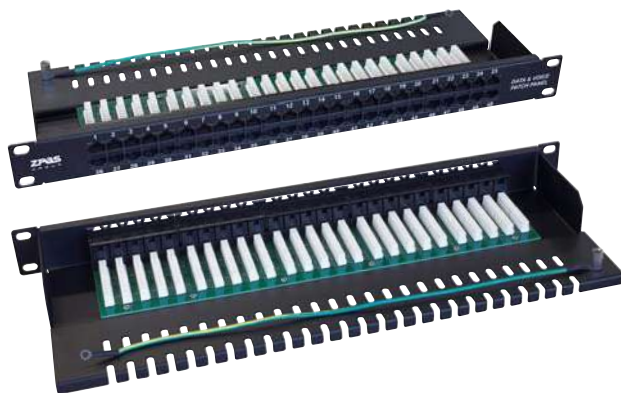
Телефонная патч-панель UTP 19" x 1 U кат. 3, 50 портов RJ45 8P6C – номер модели: T-SO-807-158
