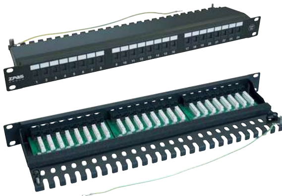
Патч-панель UTP 19" x 1 U, кат. 6 A , 24 порта черная с полкой, крышкой и пылезащитными крышками – номер модели: T-SO-806-527
