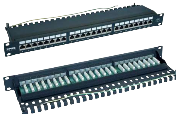
Патч-панель STP 19" x 1 U, кат. 6, 24 порта черная с полкой и крышкой – номер модели: T-SO-900-126
