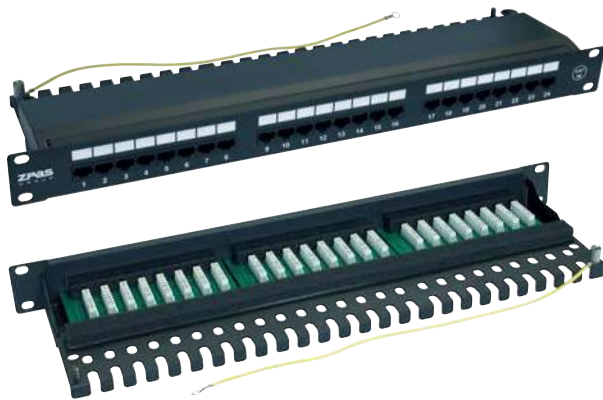
Патч-панель UTP 19" x 1 U, кат. 5e, 24 порта черная с полкой и крышкой – номер модели: T-SO-900-025
