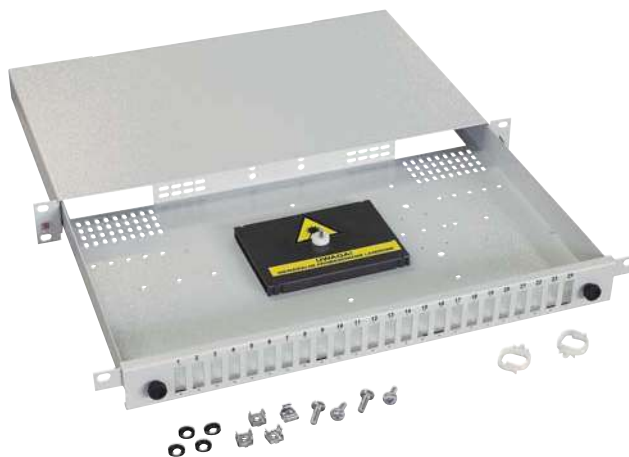
Оптический бокс OptiLAN PSP III 19/1U/24xSC duplex - номер модели: WNK-878-412
