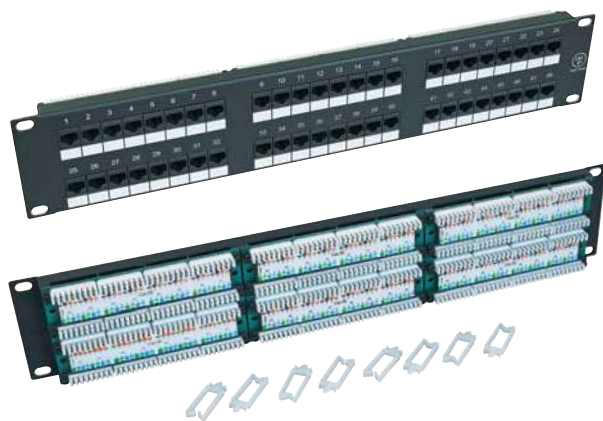
Патч-панель UTP 19" x 2 U, кат. 5e, 48 порта черная (RAL 9005) – номер модели: T-SO-900-048
