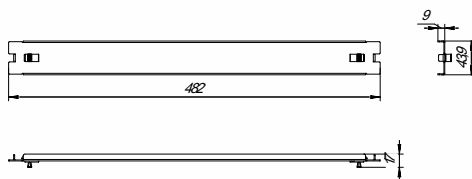
Фальш-панель 1U на защелках быст.роъем
