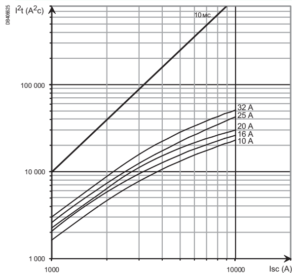
iC60 RCBO 10000 A - 2P/3P - 230 В
