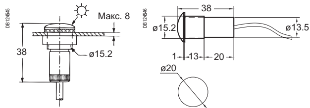
Фотоэлемент для щитового монтажа (15281) Крепится в вертикальном положении двумя винтами Ø 4 мм снаружи щита
