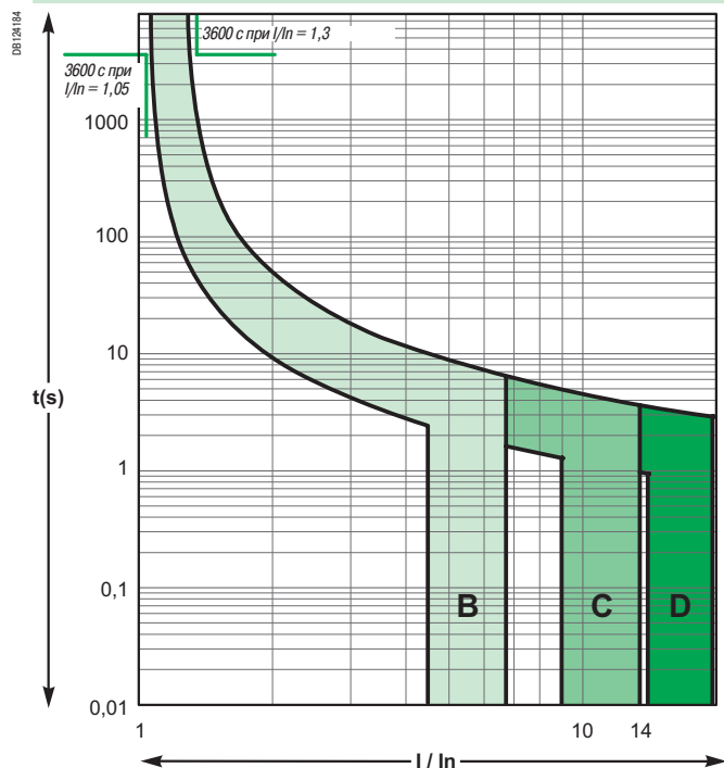
Кривые В, С, D до 4 А
