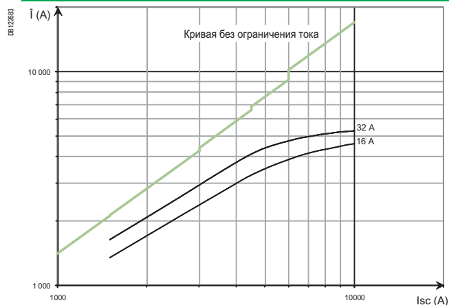
iC60 RCBO 10000 A - 2P/3P - 230 В
