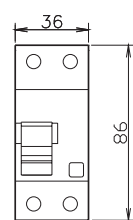
2P RCCB-ID 125 A
