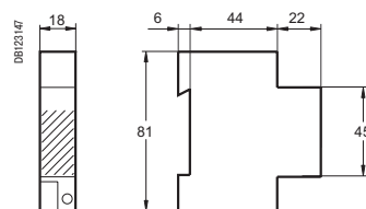
Звонок SO и зуммер iRO
