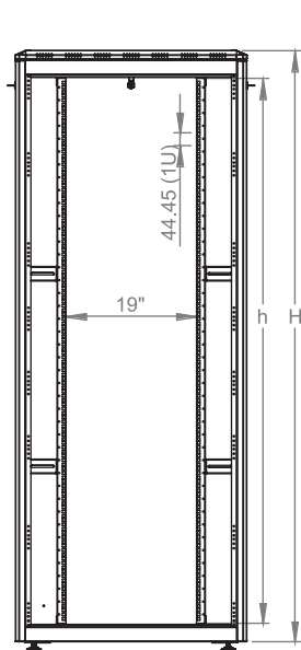
Измерения по ширине и высоте
