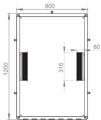
Вид сверху
