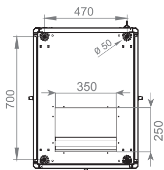
Вид снизу
