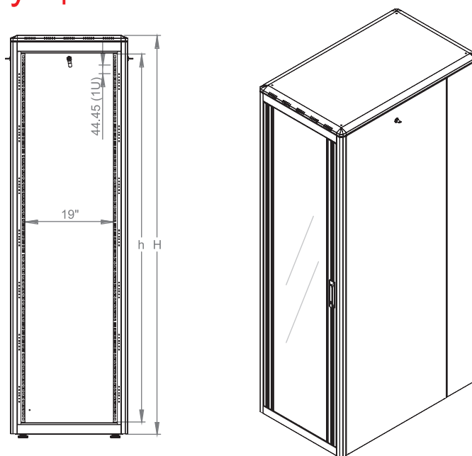
Измерения по ширине и высоте
