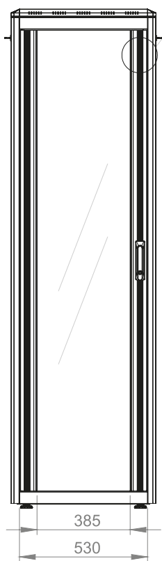
Вид спереди
