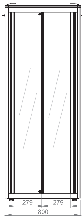
Вид спереди
