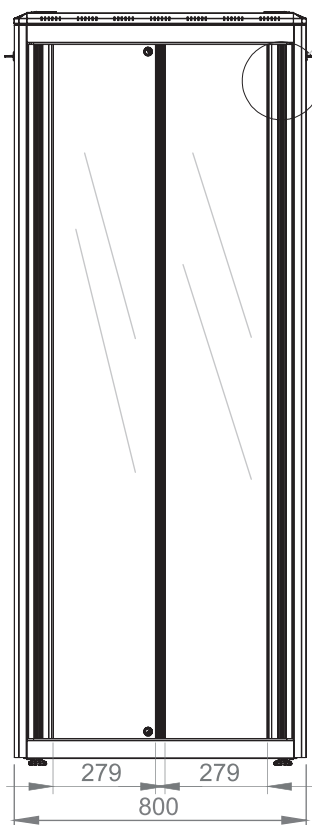
Вид спереди
