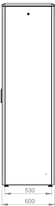
Вид сбоку
