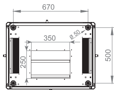
Вид снизу
