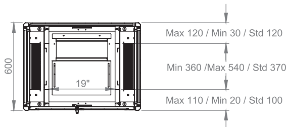
Глубина установки монтажного профиля
