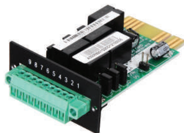
КАРТА «СУХИЕ КОНТАКТЫ» INNOVA RT 33 ID: 1180662
