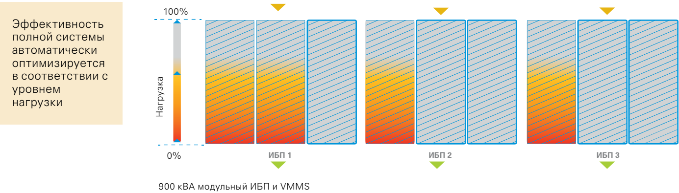
Центр обработки данных, использующий серверы с двулучевой схемой питания, ИБП Power Xpert 9395P-900 кВА в лучах А и В, нагрузка 320 кВА.
