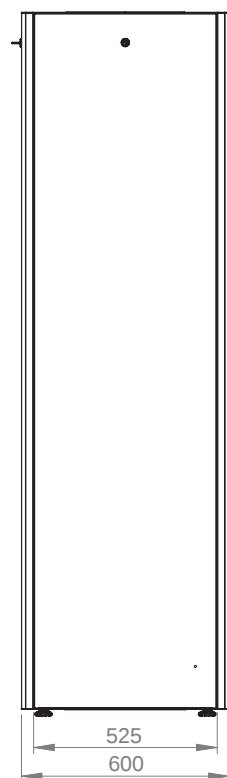
Вид сзади
