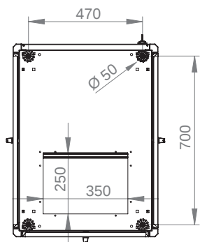
Вид снизу
