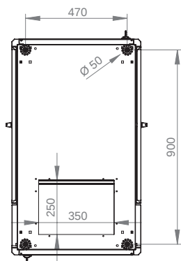
Вид снизу
