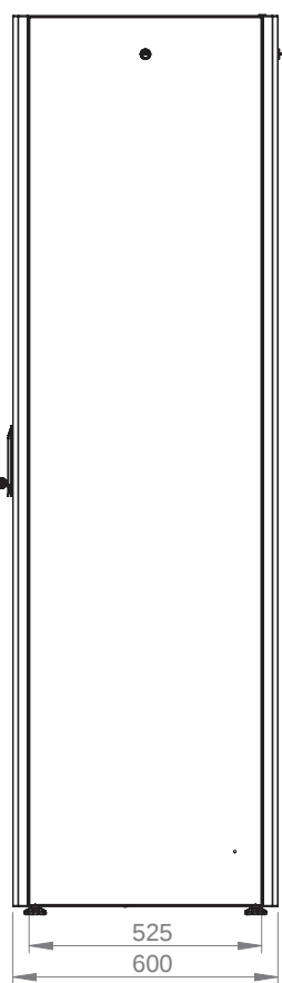
Вид сбоку
