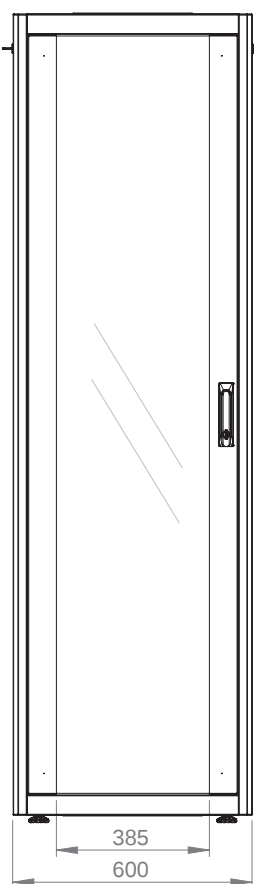
Вид спереди
