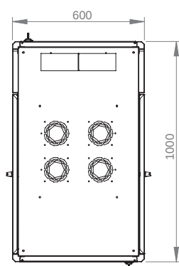
Вид сверху
