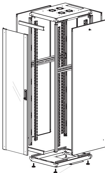
Детальный вид
