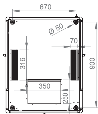
Вид сверху
