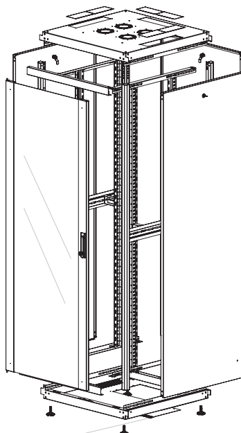
Детальный вид
