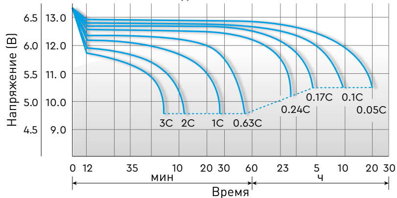
РАЗРЯДНЫЕ ХАРАКТЕРИСТИКИ
