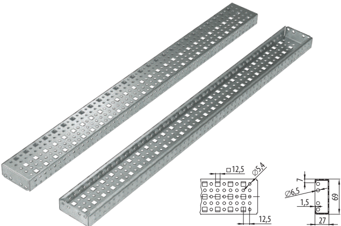
Монтажный профиль В
