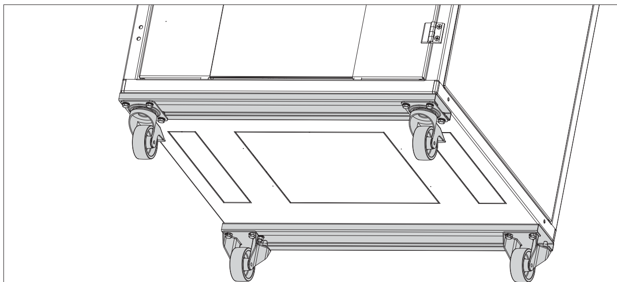
Шкаф SZB IT с установленными пластинами-адаптерами и роликами типа 300
