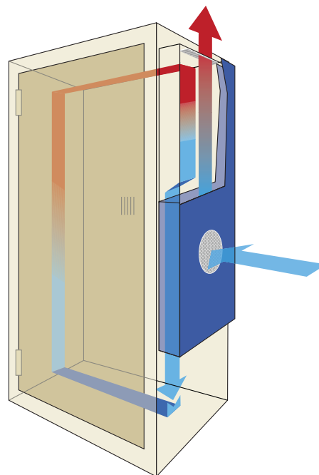
SLIM Кондиционер, устанавливаемый на двери или боковой панели шкафа. Охлаждающая мощность от 500 до 3000 Вт
