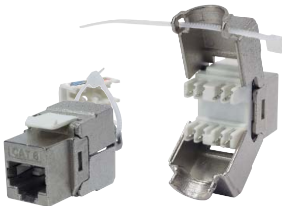
Модуль Keystone STP RJ45, категория 6 – партномер: T-SO-832-924
