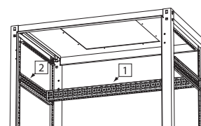
1. Монтажная рейка CLASSIC 2. Поперечная рейка CLASSIC
