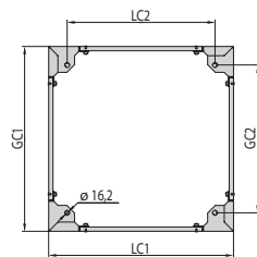
Цоколь сборный (отверстия для анкерки)
