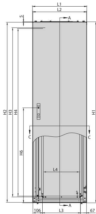
Вид спереди (шкаф с одностворчатой дверью)
