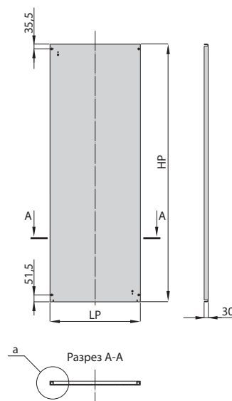
Монтажная панель
