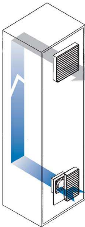
Пример вентиляции шкафа с принудительной циркуляцией воздуха
