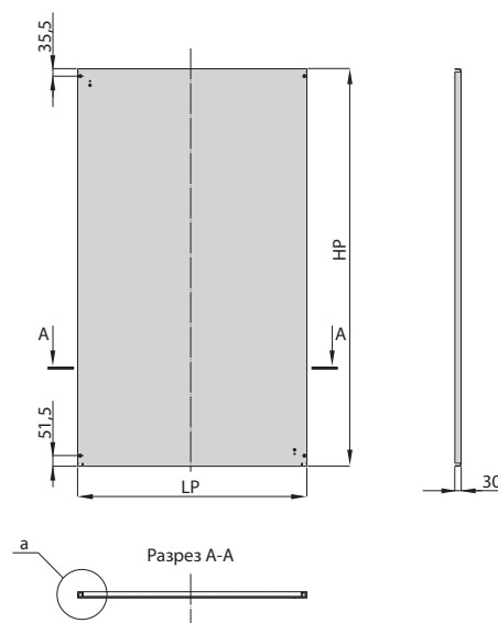
Монтажная панель
