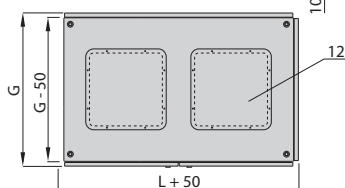
Вид сверху
