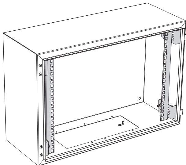
Корпус шкафа SWN с установленным комплектом 19-дюймовых уголков
