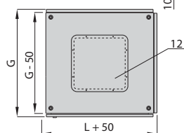
Вид сверху
