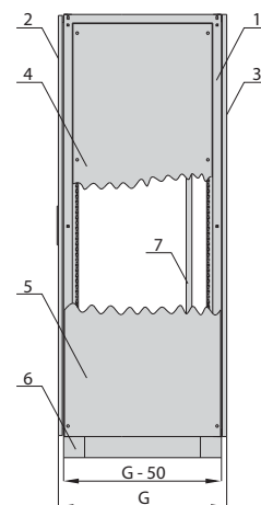
Вид с боку (сравнение вкладки и накладной боковой стенки)
