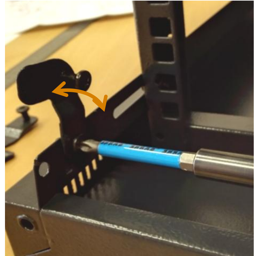
Блокираторы боковых панелей фиксируются на крыше и дне шкафа
