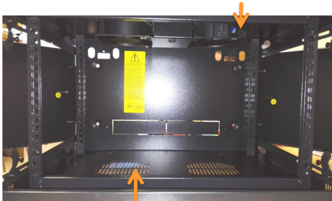
Установленный модуль вентиляторов
