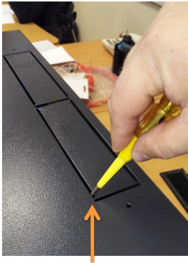
Выломав заглушки на кабельном вводе
