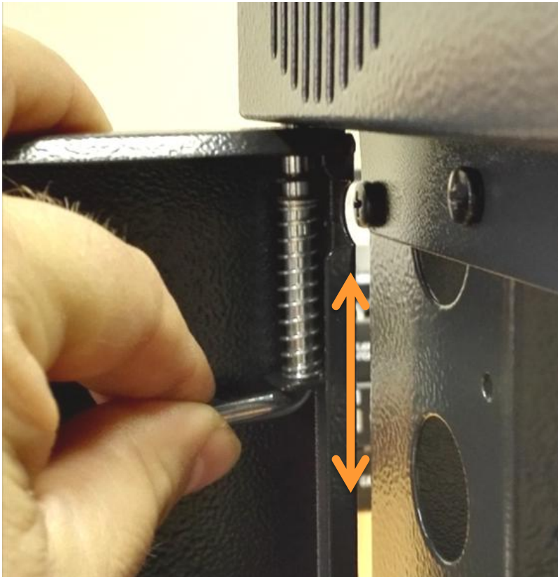
Боковые панели устанавливаются на шпингалеты
