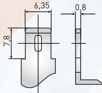
Нож F2
