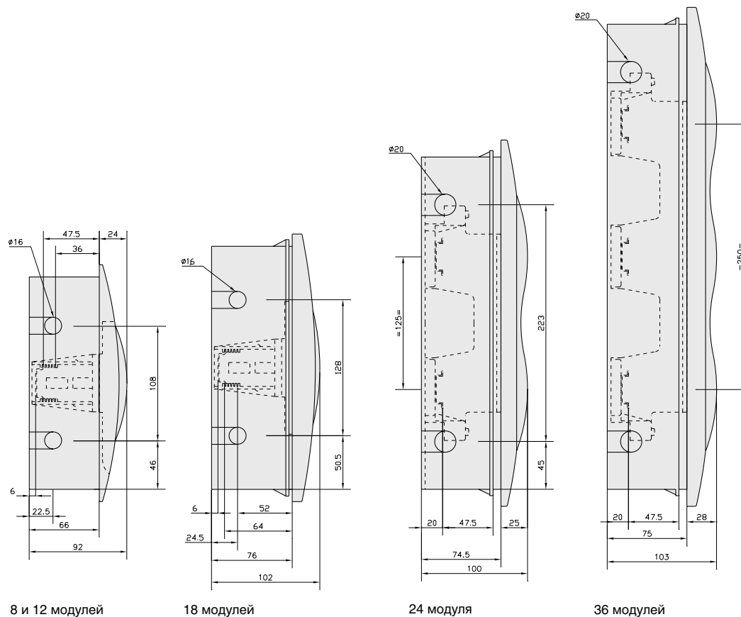
8 и 12 модулей
