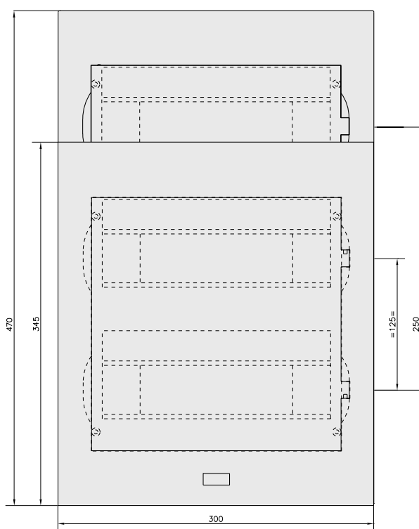
24 и 36 модулей
