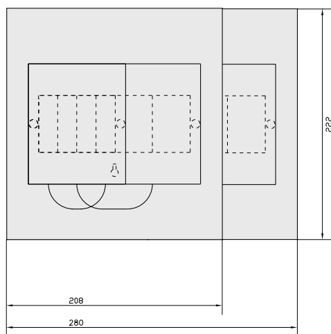
8 и 12 модулей
